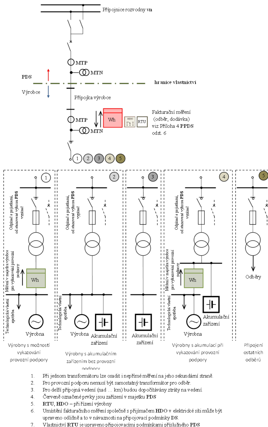
Obr. 24 Připojení výrobní a akumulčního zařízení samostatným vedením do vn rozvodny DS
