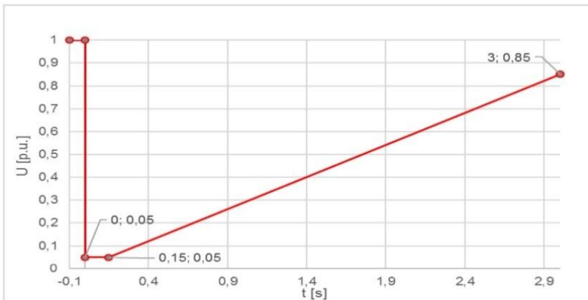
Obrázek č. 3 Autonomní charakteristika FRT pro nesynchronní VM A1, A2, B2, C
