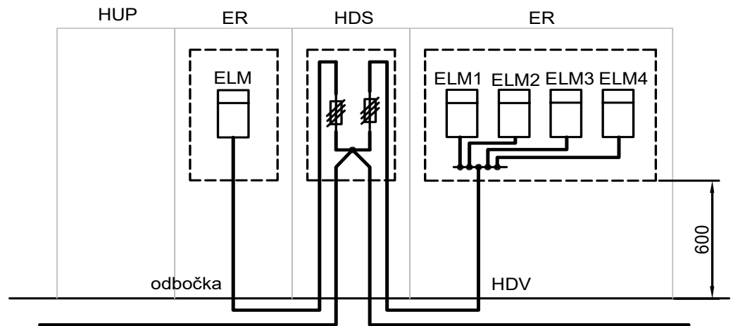
Umístění HDS – připojení z kabelového vedení, více sad pojistek
