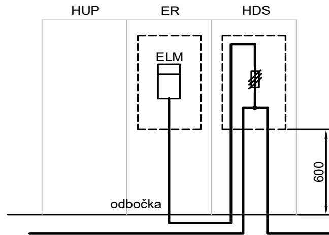
Umístění HDS – připojení z kabelového vedení
