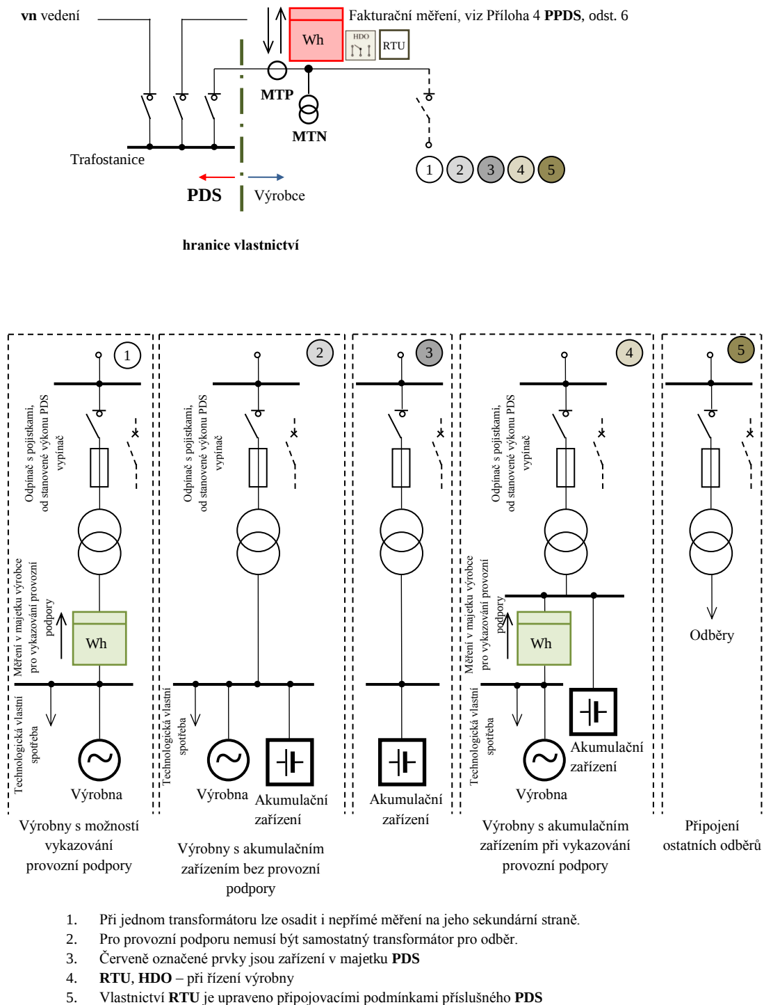
Obr. 19 Připojení výroby a akumulčního zařízení zasmyčkováním do vn vedení DS
