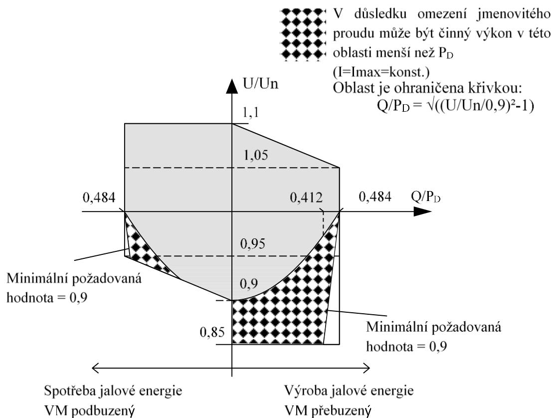
Obr. 2 Jalový výkon VM A1 pro P=P_D
