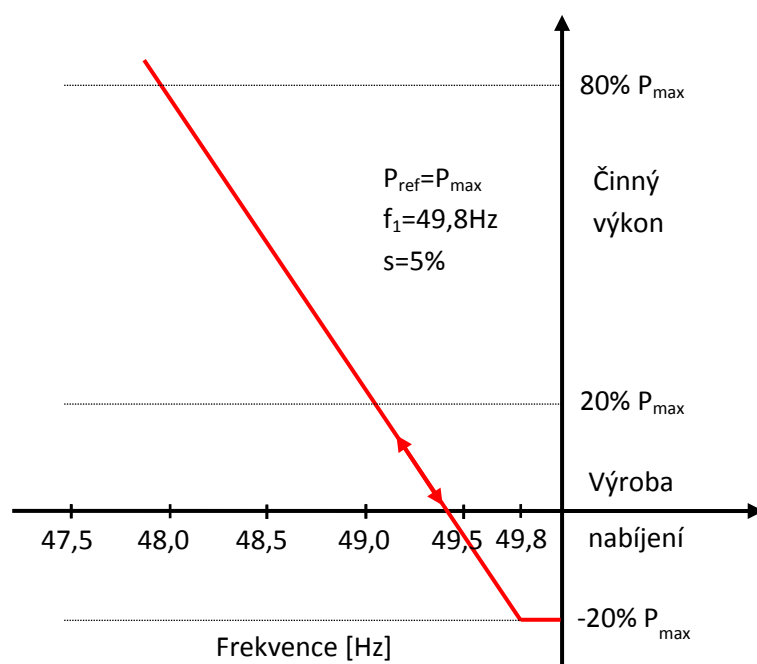
Obr. 12 Frekvenční odezva činného výkonu na podfrekvenci u akumulačního zařízení.
