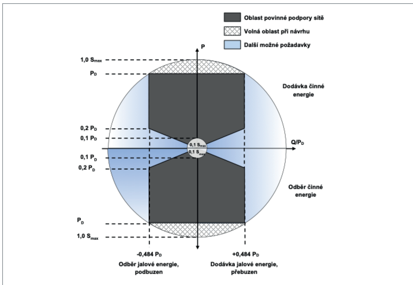
Obr. 6.11.1: Rozsah podpory nadpětí jalovým výkonem
