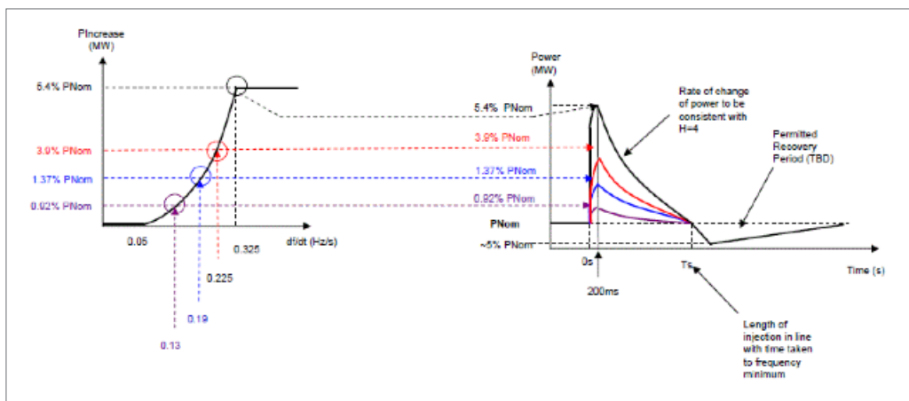
Obrázek 2 - Ilustrativní znázornění změny činného výkonu pro umělou setrvačnost
