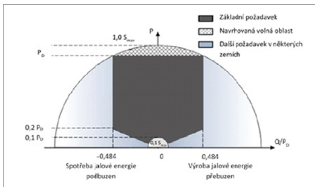
Obrázek 2 – Rozsah podpory nadpětí jalovým výkonem
