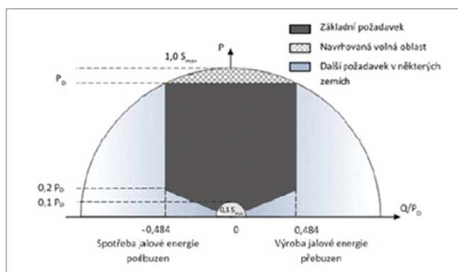
Obrázek 1 – Rozsah podpory napětí jalovým výkonem
