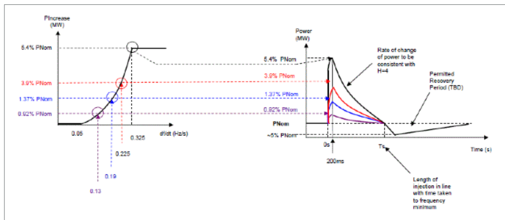
Obrázek 6.14.4 - Ilustrativní znázornění změny činného výkonu pro umělou setrvačnost
