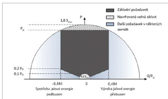
Obrázek 6.12.1 – Rozsah podpory napětí jalovým výkonem
