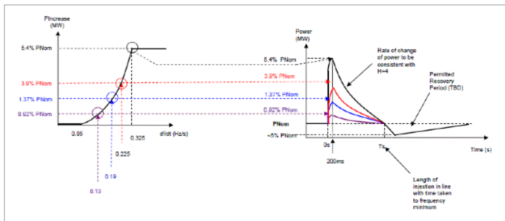
Obrázek 6.14.4 - Ilustrativní znázornění změny činného výkonu pro umělou setrvačnost
